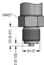
G1/2" EN 837
